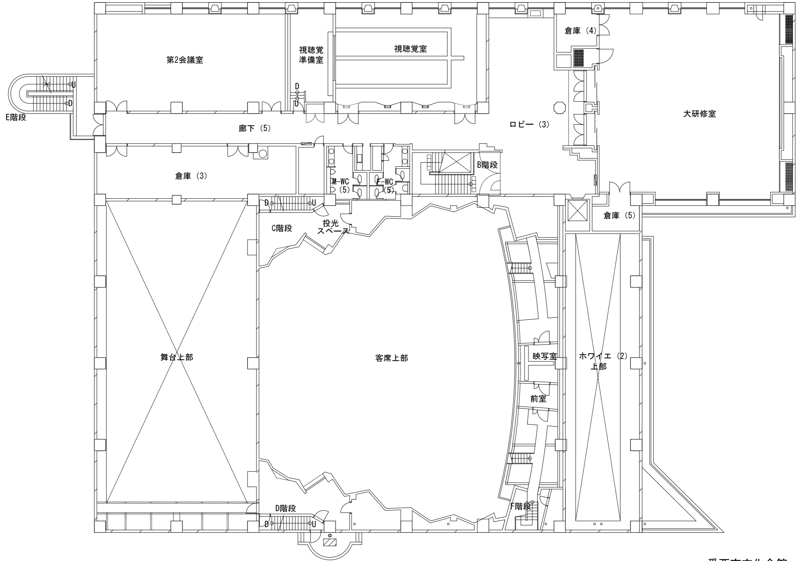
愛西市文化会館 3階平面図
