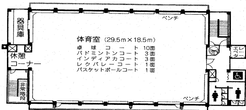
3階平面図
