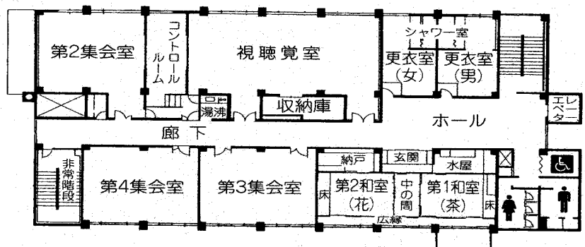
2階平面図
